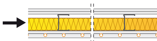
mit Variotherm ModulPlatte
