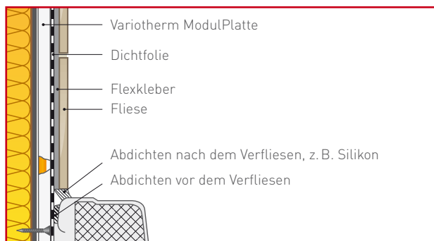
▲ Anschlüsse von Dusch- bzw. Badewannen
