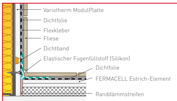
▲ Wand-Estrichbildung im wasserbeanspruchten Bereich
