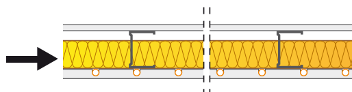
mit Variotherm ModulPlatte
