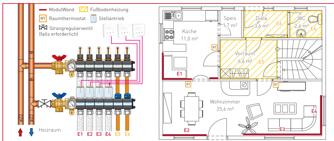
▲ Kombination von Heizsystemen, Beispiel Einfamilienhaus (Erdgeschoß)
